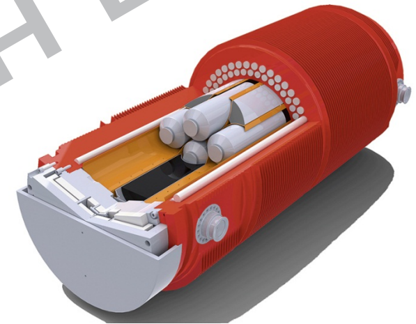
Schnittzeichnung Transportbehälter vom Typ B – Gewicht: viele Tonnen
