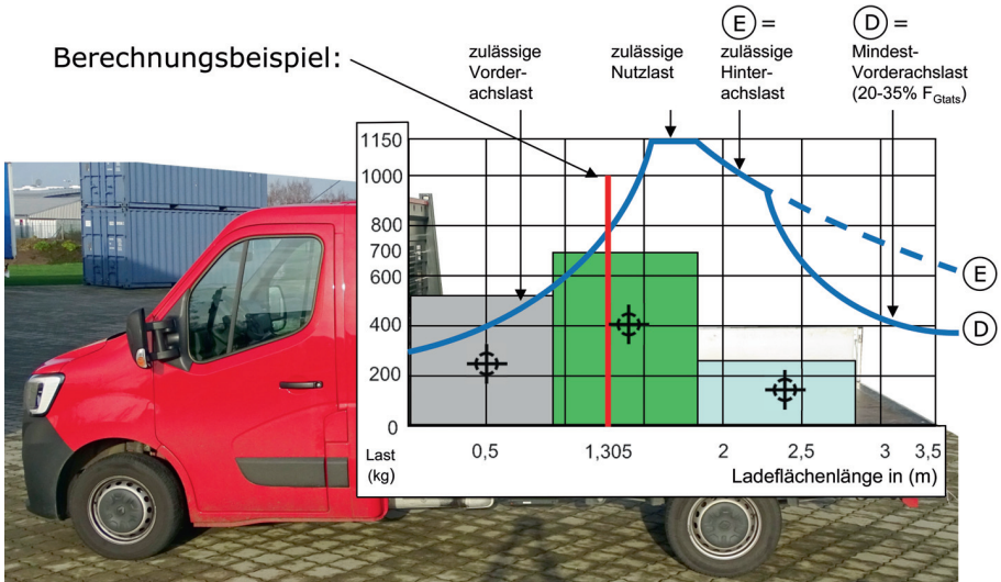
Bild 3.28: Lastverteilungsplan zum Berechnungsbeispiel
