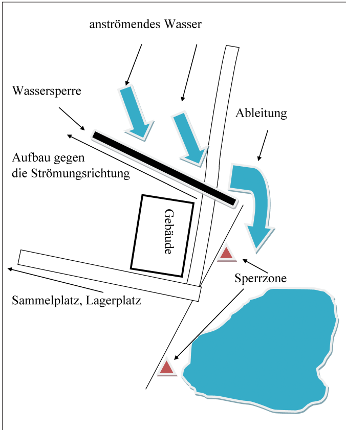
Ableitung anströmenden Wassers (schematische Darstellung)
