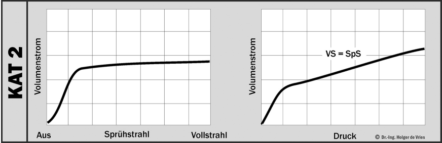
Abbildung 26: Typische Kennlinien eines Strahlrohrs mit variabler Strahlform bei konstantem Volumenstrom
