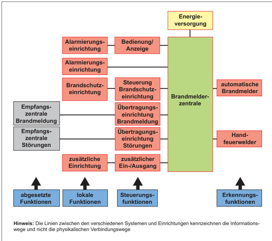
Abbildung 2: Brandmeldeanlage mit den im Zusammenhang stehenden Systemen und Einrichtungen (Quelle: Hans Kemper, Geseko)
