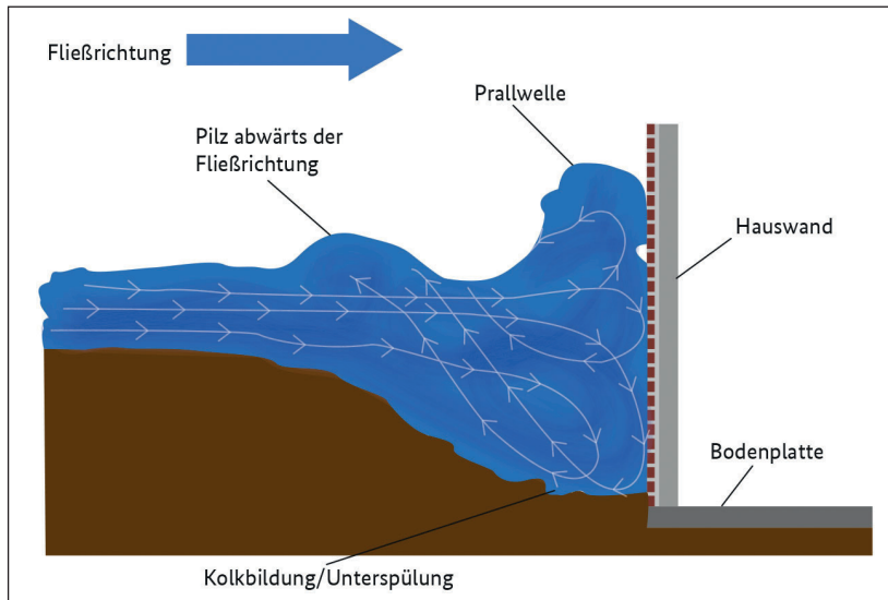
Abb. 10: Fließverhalten einer Prallwelle (Grafik: THW-Ltg. Nadine Bottin)
